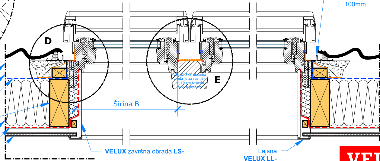
Odjeljak B-B / M10
